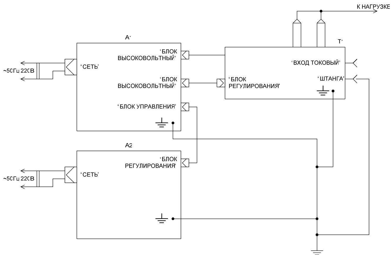
Рис. 2. Схема соединения блоков установки.
