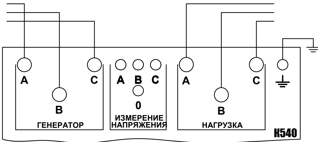
Рис. 2. Непосредственное измерение силы тока в однофазной сети.
