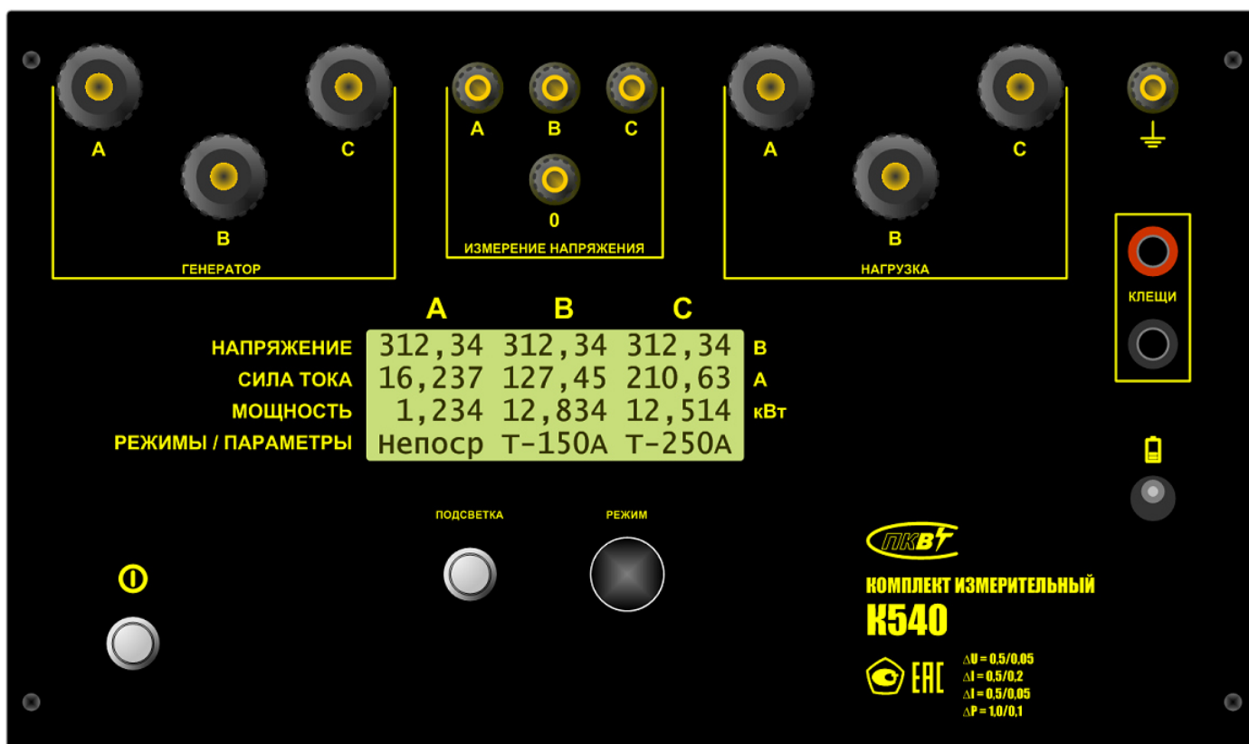
Рис. 1. Внешний вид передней панели комплекта К540.
