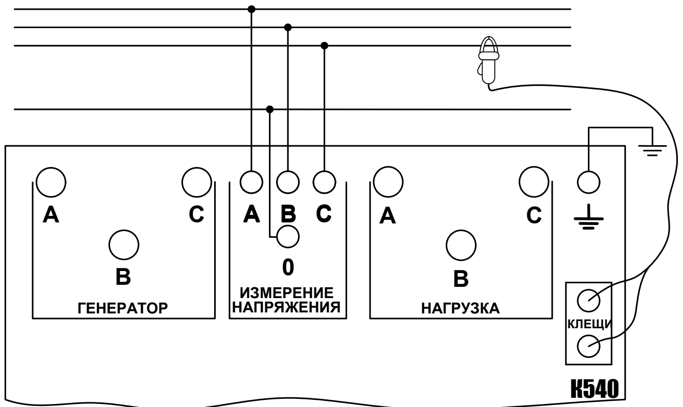
Рис. 4. Непосредственное измерение силы тока в четырёхпроводной трёхфазной сети.
